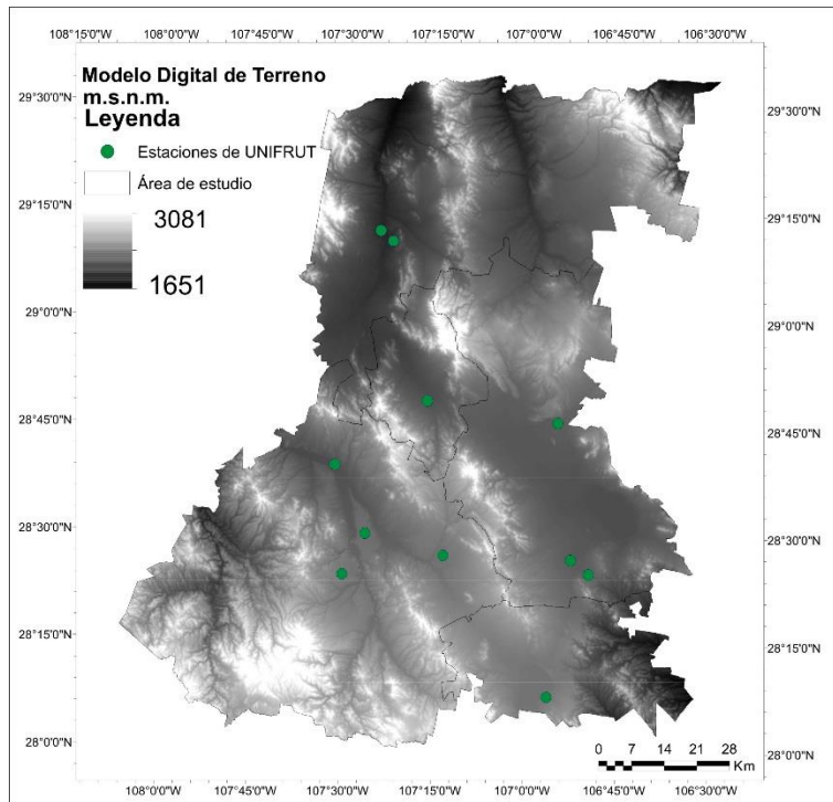
Figura 2. Modelo digital de elevaciones (m.s.n.m.)
