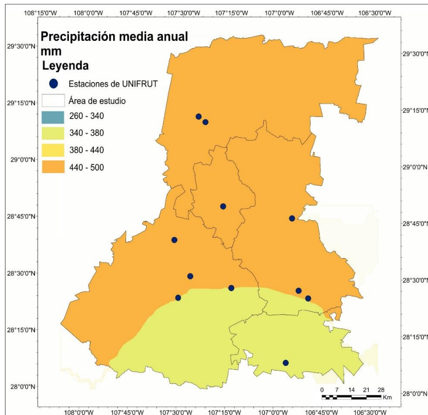
Figura 4. Precipitación media anual (PMA; mm)
